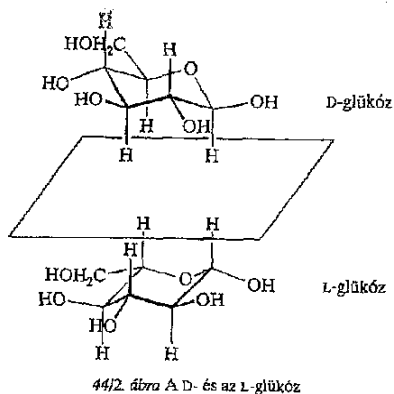
44/2. ábra A D- és az L-glükóz
